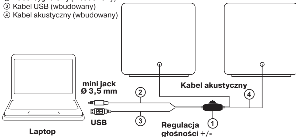
Rys. 1. Schemat połączenia
